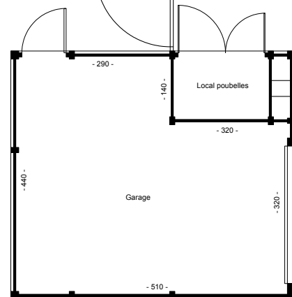
PLAN RDC
