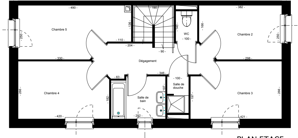
PLAN ETAGE
